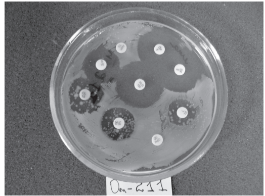
Рис. 2. Верифікація ізоляту № 211, виділеного з агроecosистеми Inula helenium
