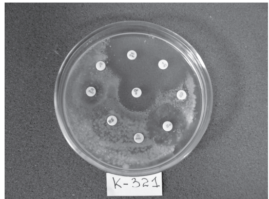
Рис. 3. Верифікація ізоляту № 321, виділеного з агроecosистеми Calendula officinalis
