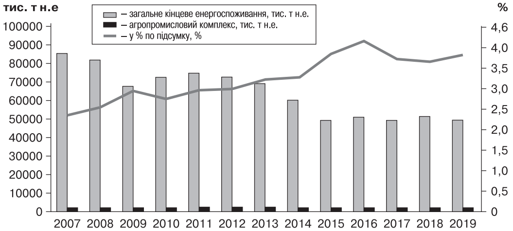
Рис. 1. Кінцеве енергоспоживання за 2007–2019 рр.
