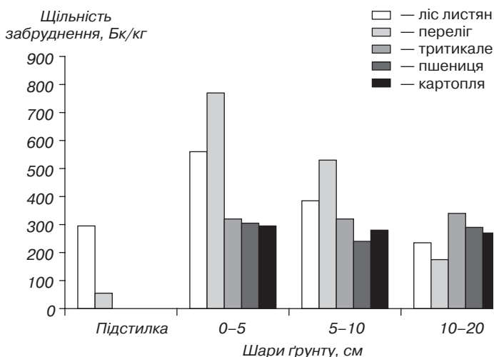
Рис. 1. Розподіл питомої активності ^{137}\text{Cs} у профілі дерново-підзолистого ґрунту в агроценозах і природних екосистемах
